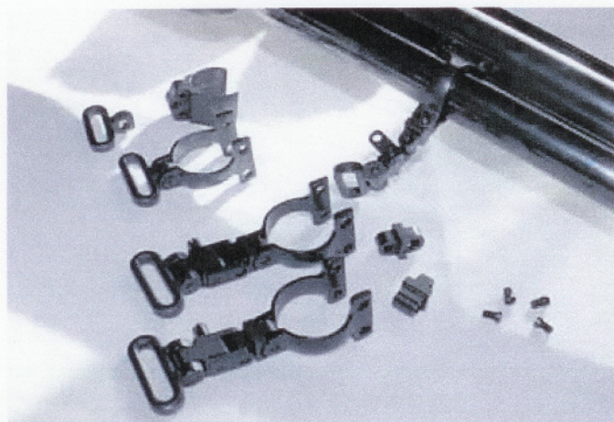
Abnehmbare Riemenbügel von Recknagel. (Foto: Michele Costantini)
